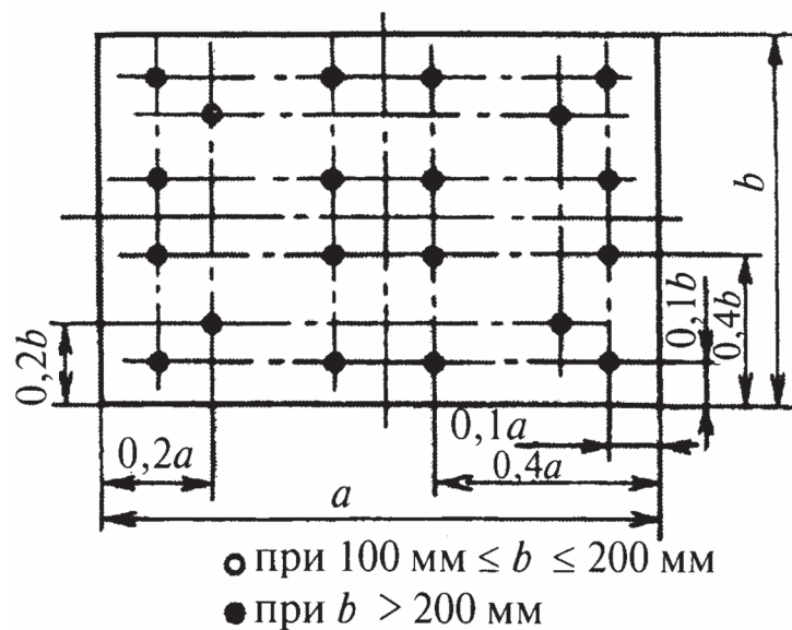
Рисунок 2 – Координаты точек измерения давлений и скоростей в воздуховодах прямоугольного сечения
